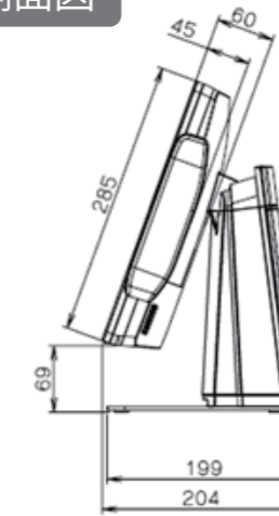
側面図
